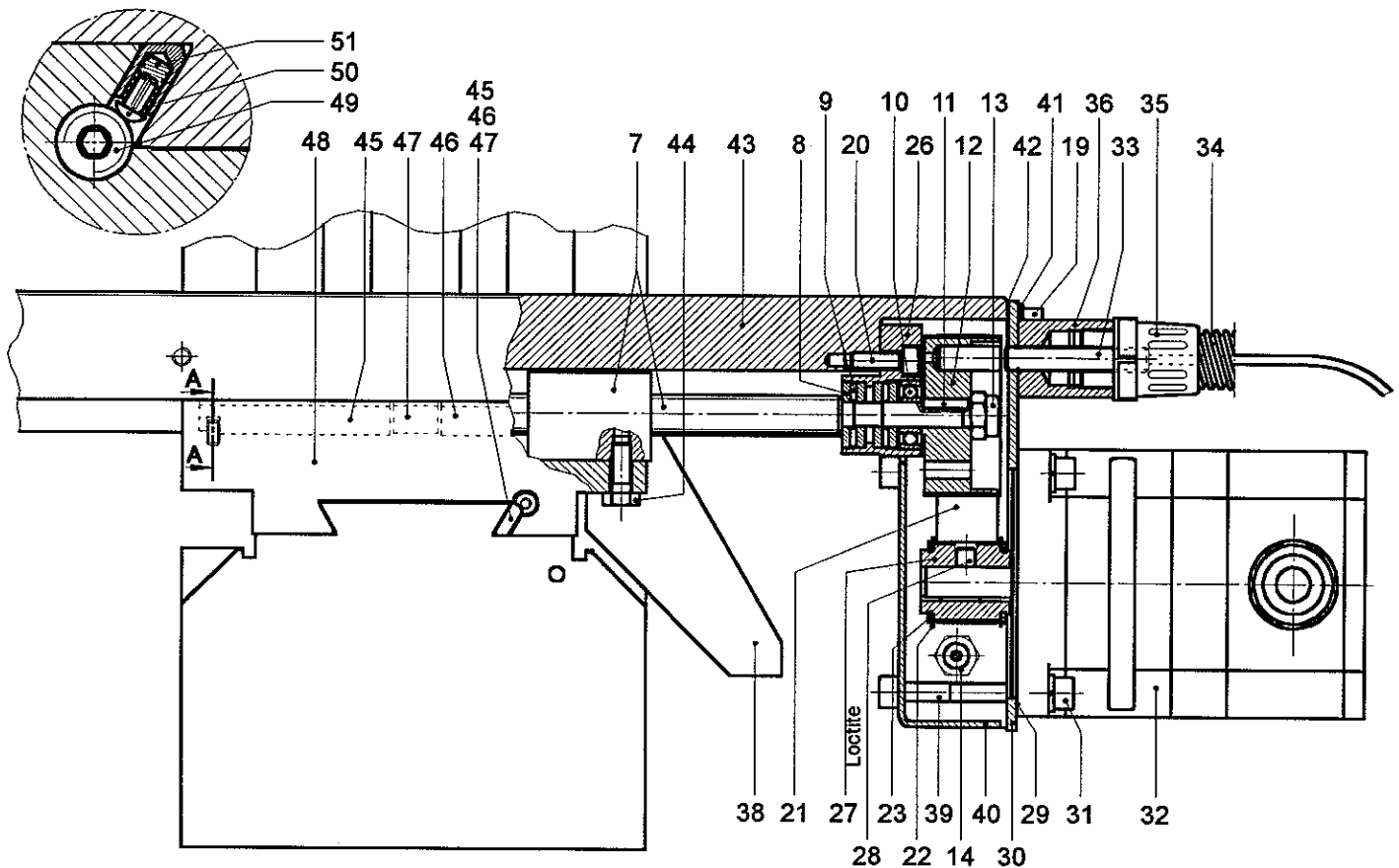
Schnitt A-A
